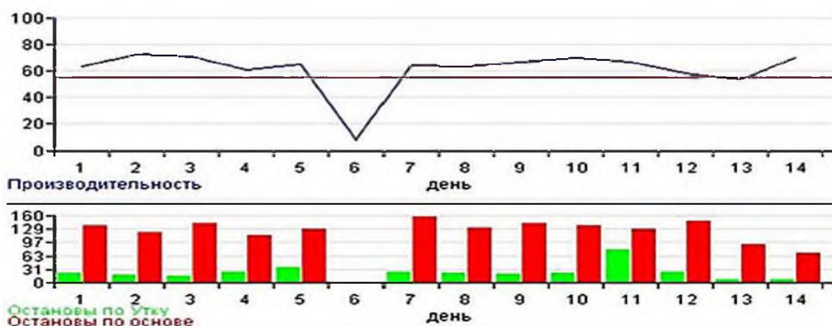
Рисунок 3 – График производительности ткацкого станка и гистограмма обрывности при использовании в шликте препарата Аркофил PPL Figure 3 – Loom performance graph and breakage histogram when using Arcofil PPL in sizing
